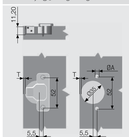
راهنما سوراخ‌کاری برای لولا با فاصله آکس تا آکس ۵۲ میلی‌متر
