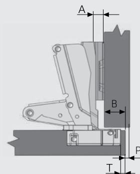
پایه لولا
