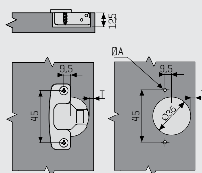
ابعاد سوراخ‌کاری A (میلی‌متر):
