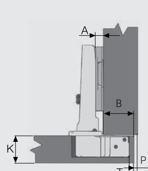
روکار
