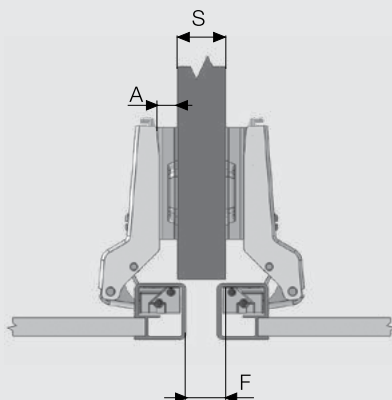
نیم‌ونیم با طول خم ۹ میلی‌متر
