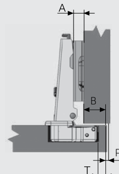
پایه لولا
