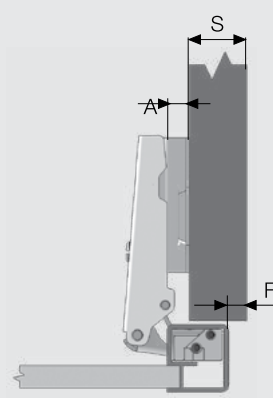
روکار
