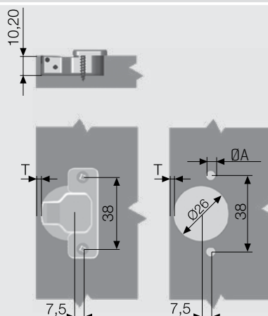
راهنما سوراخ‌کاری برای لولا با فاصله آکس تا آکس ۳۸ میلی‌متر
