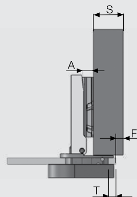
روکار
