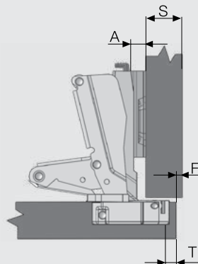
پایه لولا
