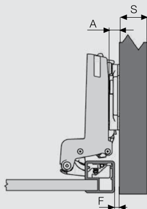
توکار با طول خم ۱۸ میلی‌متر
