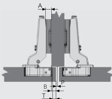
پایه لولا
