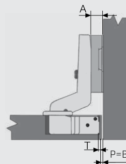
روکار
