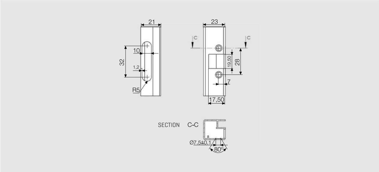
ابعاد سوراخ کاری
