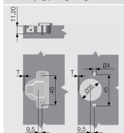
راهنما سوراخ‌کاری برای لولا با فاصله آکس تا آکس ۴۵ میلی‌متر
