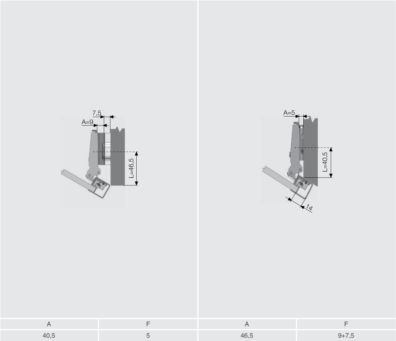
ابعاد سوراخ کاری
