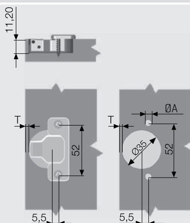
راهنما سوراخ‌کاری برای لولا با فاصله آکس تا آکس ۵۲ میلی‌متر
