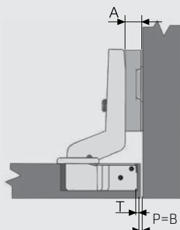
توکار با طول خم ۱۶ میلی‌متر
