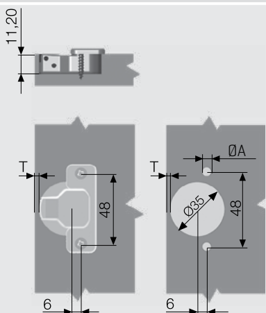
راهنما سوراخ‌کاری برای لولا با فاصله آکس تا آکس ۴۸ میلی‌متر
