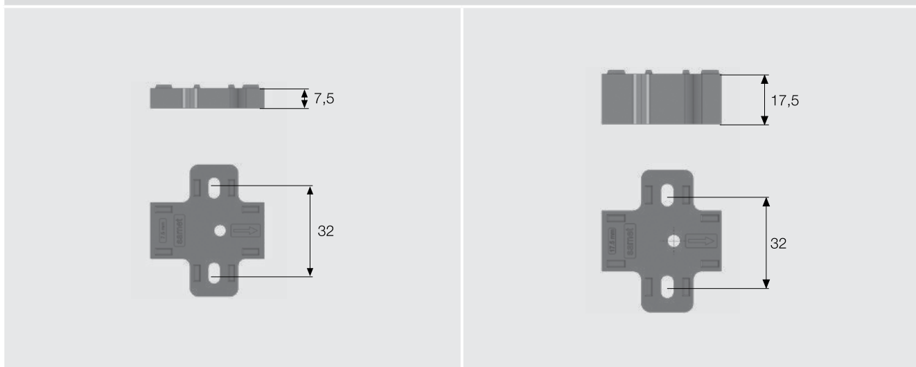
ابعاد
