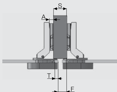
نیم‌ونیم با طول خم ۹ میلی‌متر
