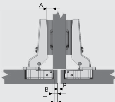
نیم‌ونیم با طول خم ۹ میلی‌متر
