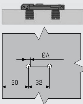
نوع نصب کاپ لولا
