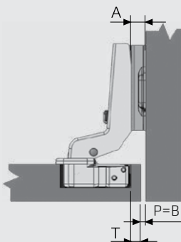
توکار با طول خم ۱۸ میلی‌متر
