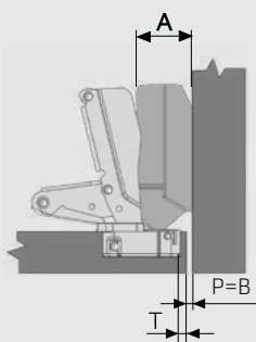
پایه لولا
