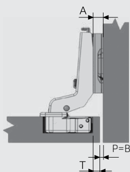
پایه لولا
