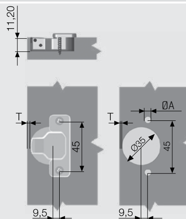
راهنما سوراخ‌کاری برای لولا با فاصله آکس تا آکس ۴۵ میلی‌متر
