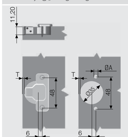
راهنما سوراخ‌کاری برای لولا با فاصله آکس تا آکس ۴۸ میلی‌متر
