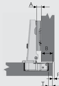
روکار
